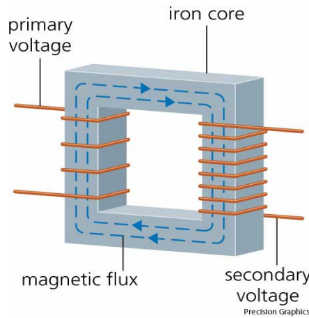
Şekil 7 Transformatör
